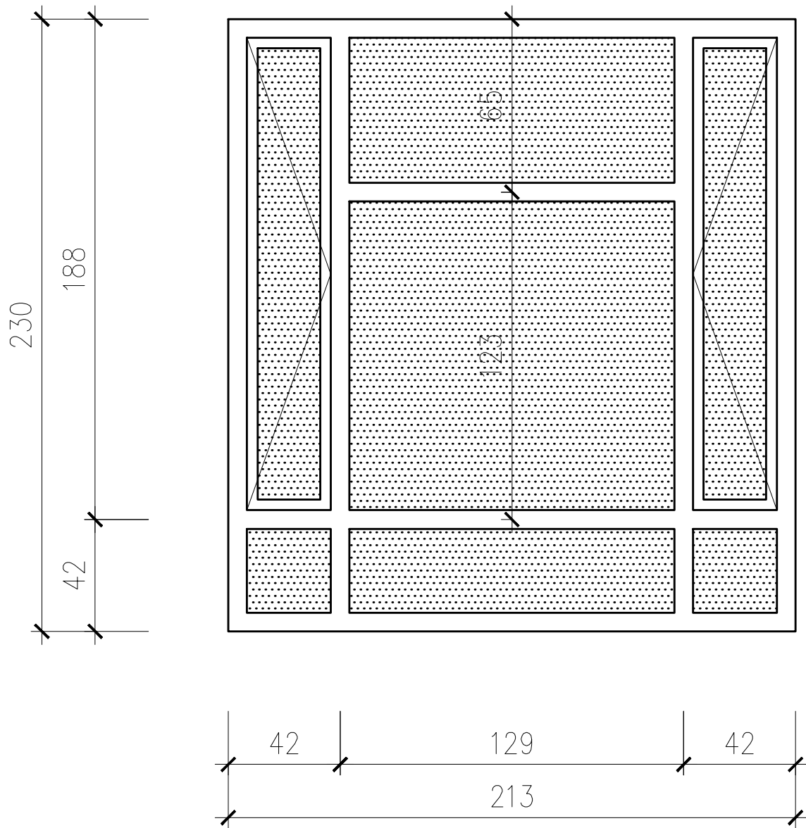
Прозорец на ул. "Сердика" 6-8 2 бр.
